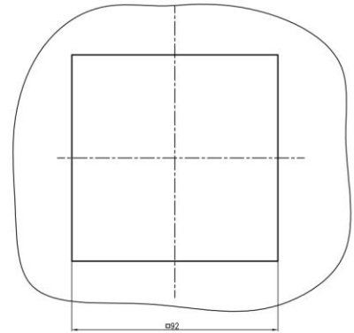
Einbauausschnitt
