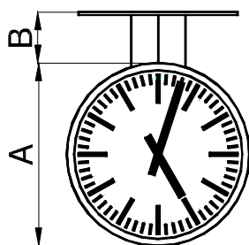
dvostranska izvedba – pritrjitev na strop ali steno
